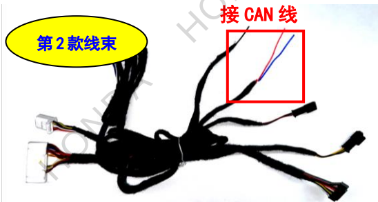
第 2 款线束 CAN 线颜色为：蓝色&粉色
