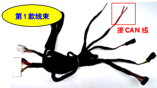
第 1 款线束 CAN 线颜色为：橙色&橙棕色
