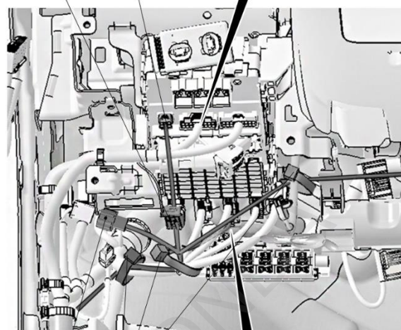
【保险丝盒下部视图】
