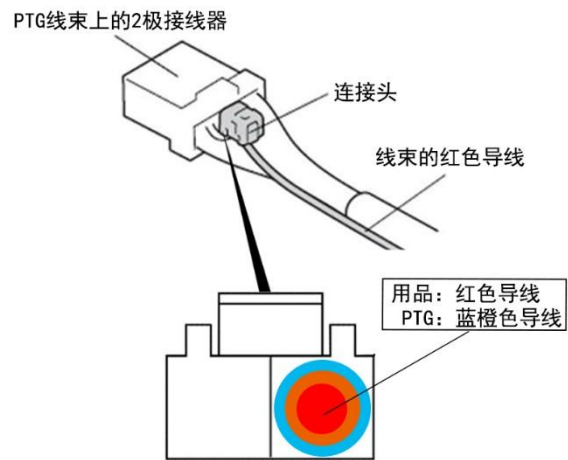
【线束侧视图】
