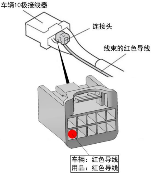
【线束侧视图】
