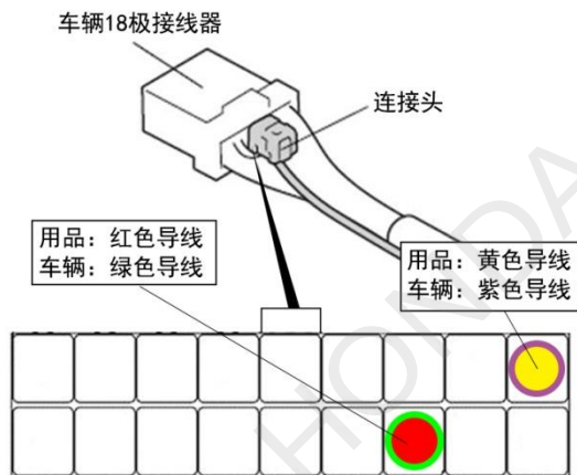
【线束侧视图】
