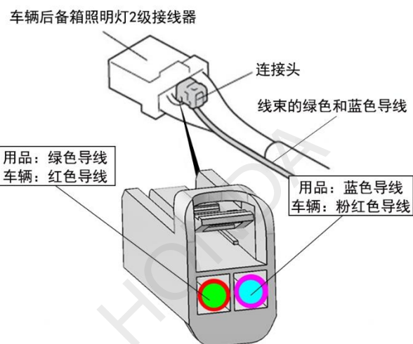
【线束侧视图】
