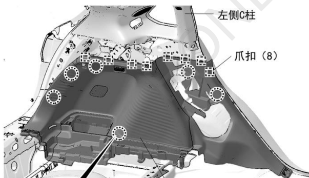
尾箱左侧内衬板
