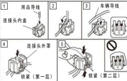
【线束侧视图】
