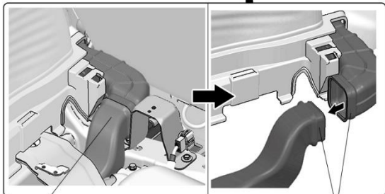
尾箱电池通风管
