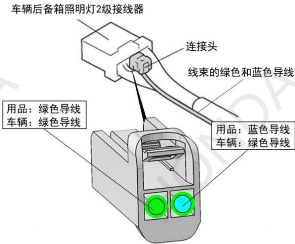
【线束侧视图】
