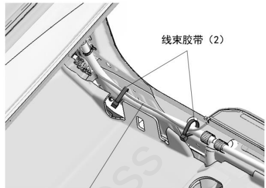
右前流光踏板的线束
