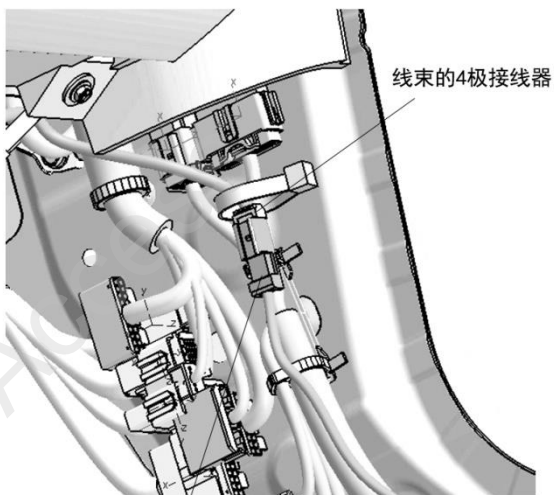
右前流光踏板的4极接线器
