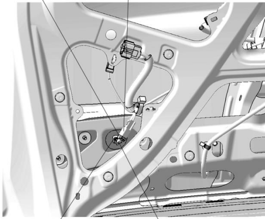
左尾灯的8极接线器 线束的8极接线器 插入左尾灯的8极接线器
