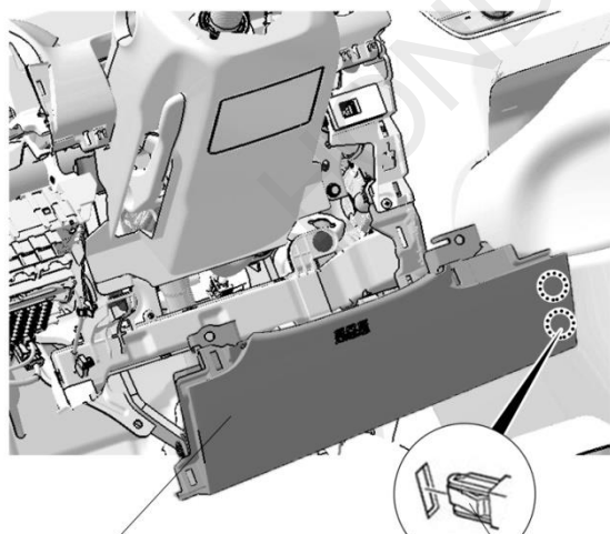
驾驶席膝部安全气囊组件
