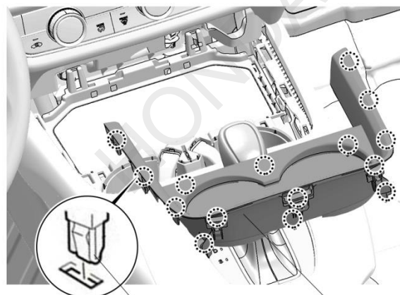
水杯座饰件
