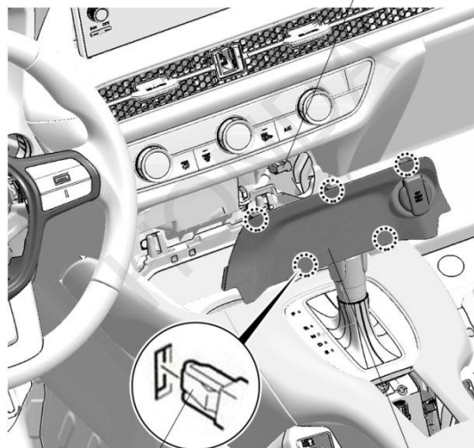
夹扣 (5)
