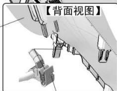
驾驶席下护板
