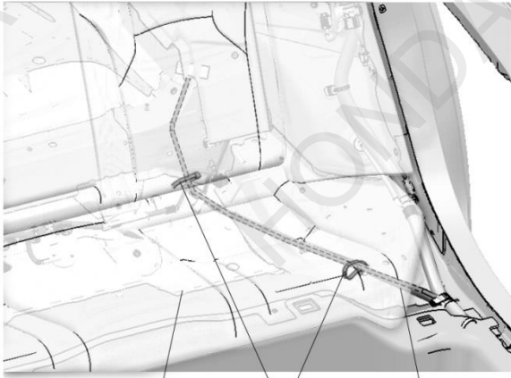
后排座垫 拉起 线束胶带 (2) 车辆线束
