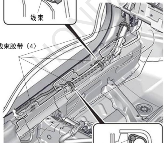
线束 线束胶带 车辆线束 地板地毯 车辆面板
