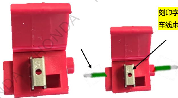
适用 0.13-0.3 线径
