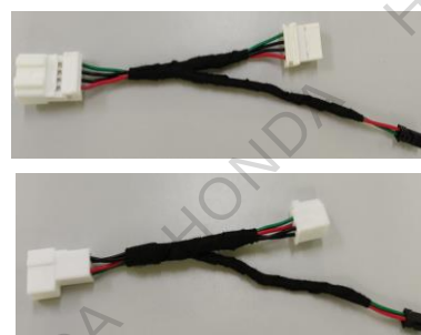
刹车开关线束(2 选 1)
