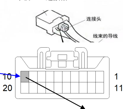
车辆 20P 连接器
