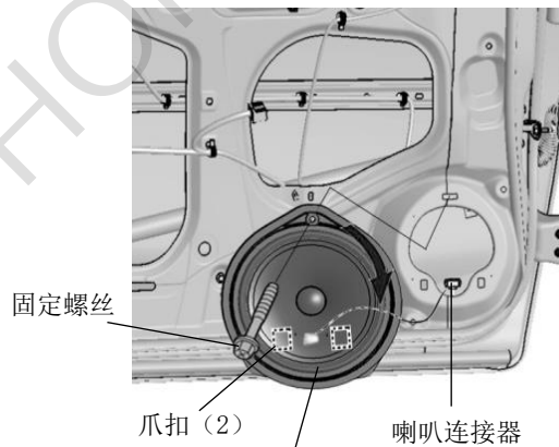
Stage3 607CF中低音喇叭 (含专用组件)
