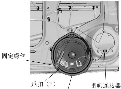
Stage3 627F同轴喇叭 (含专用件)
