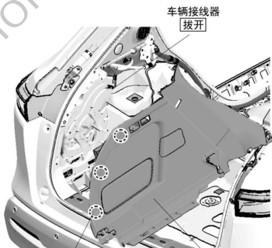
夹扣 (3)
