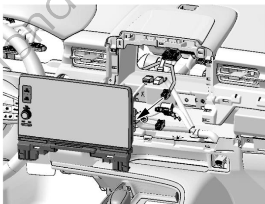
线束A接线器的 连接位置
