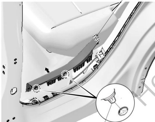
夹扣 (2)
