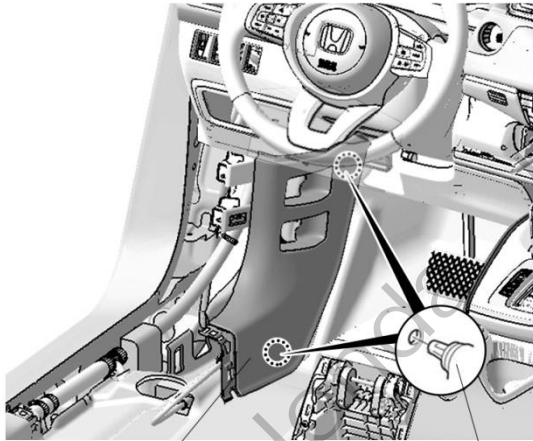
左前侧饰板
