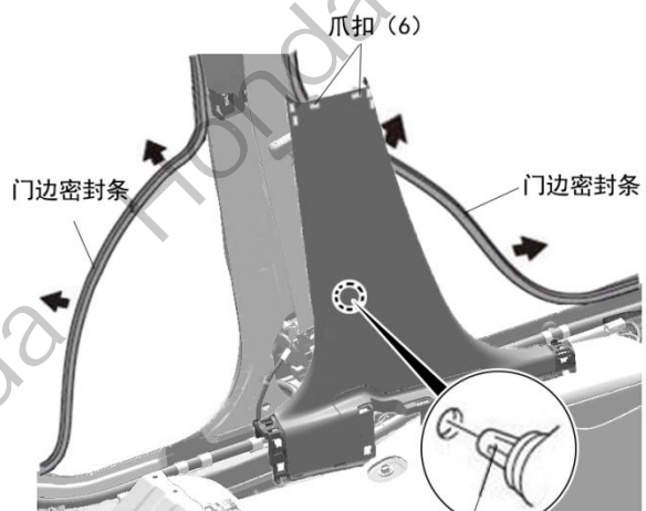
夹扣
