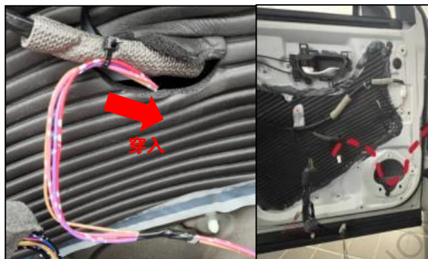
完整的走线图
