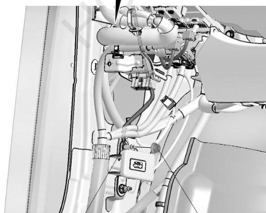
线束的地线端子
