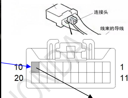
车辆 20P 连接器
