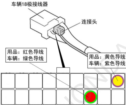
【线束侧视图】
