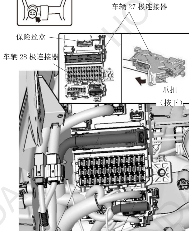
车辆 27 极连接器 车辆 28 极连接器
