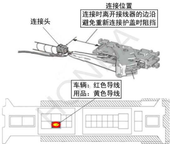
【线束侧视图】
