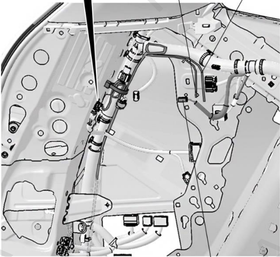
原车后备箱照明灯的 2级接线器
