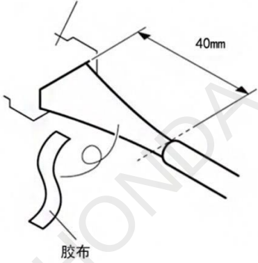
后备箱照明灯2级接线器
