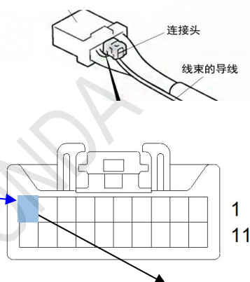
车辆 20P 连接器
