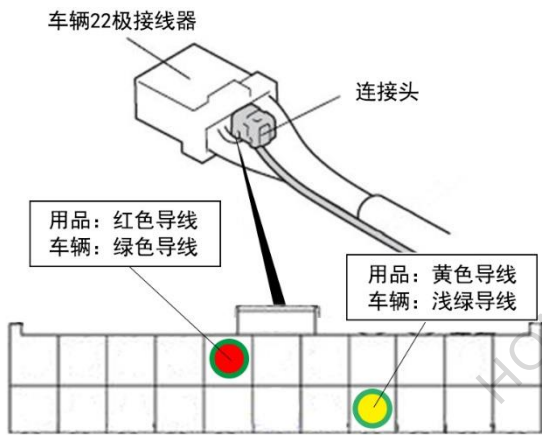
【线束侧视图】
