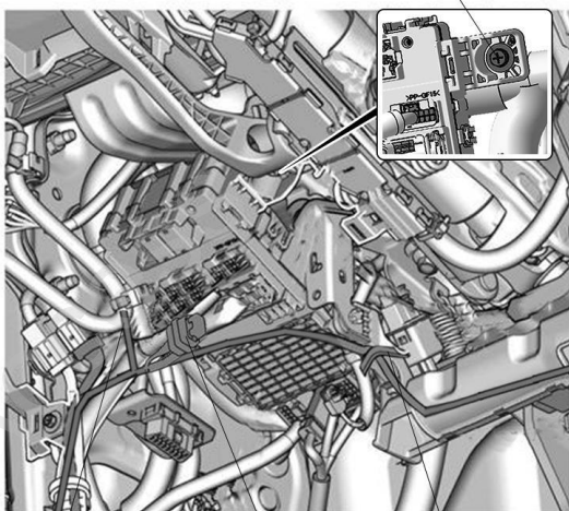
螺栓 拆出 线束A的红色导线 线束A的30A 保险丝 线束胶带
