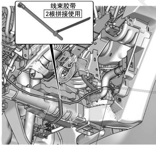
线束胶带 2根拼接使用 驾驶席脚部风管 线束胶带
