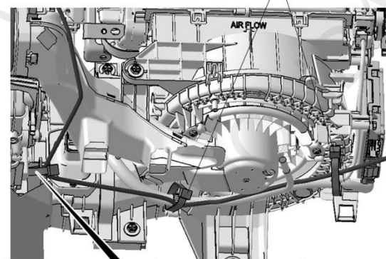
线束胶带 (2)
