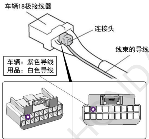
【线束侧视图】
