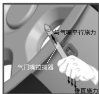
3. 使用气门嘴拉拔器 安装传感器总成
